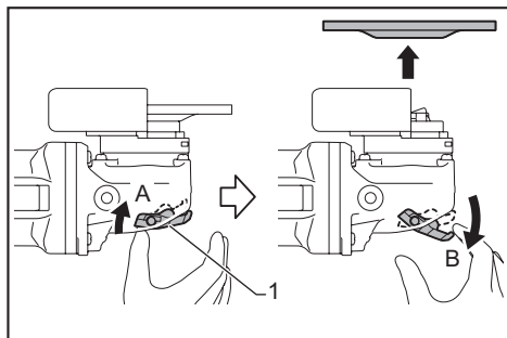
► 1. Release lever
